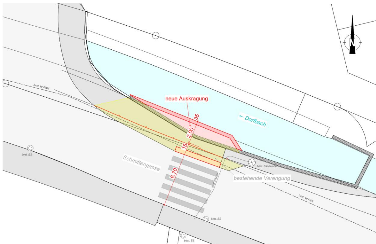
Abbildung 2: Situation der vorgesehenen Auskragung
