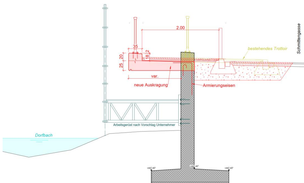
Abbildung 1: Querschnitt durch die bestehende Stützmauer und die neue Auskragung
